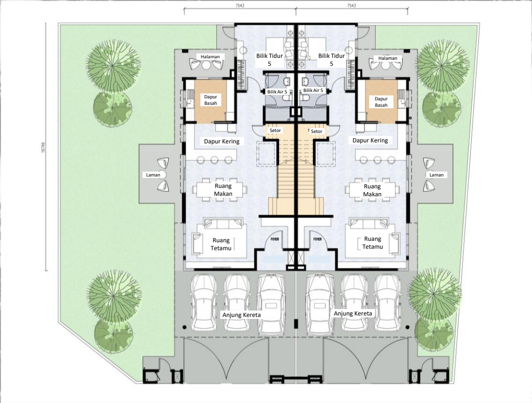
Pelan Tingkat Bawah
