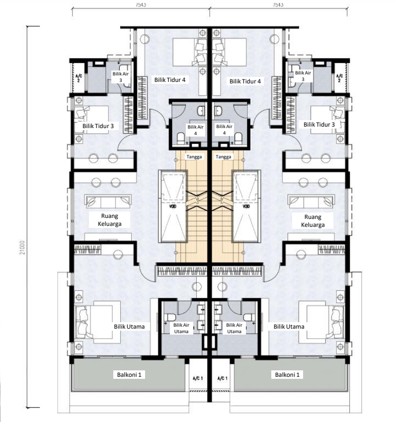
Pelan Tingkat Satu
