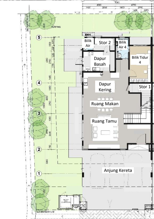
Pelan Tingkat Satu
