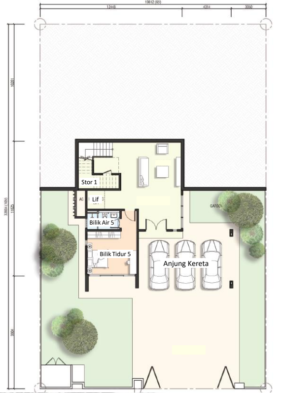
Pelan Tingkat Bawah
