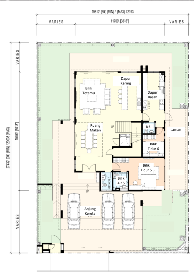
Pelan Tingkat Bawah
