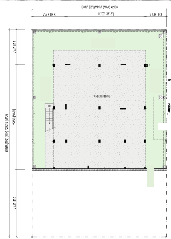
Pelan Separa Bawah Tanah
