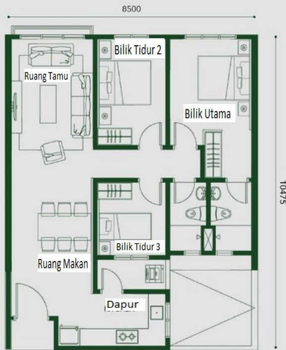
850 TYPE B K.P (Juliet Balkoni)
