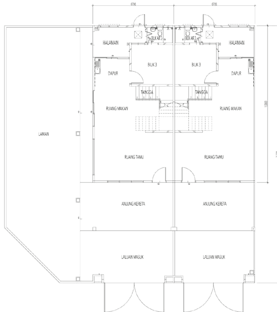
PELAN TINGKAT BAWAH
