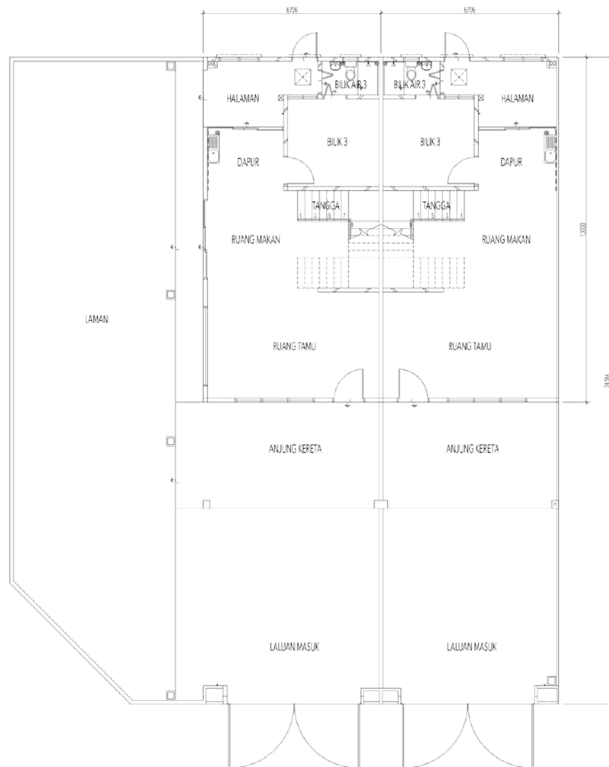
PELAN TINGKAT BAWAH
