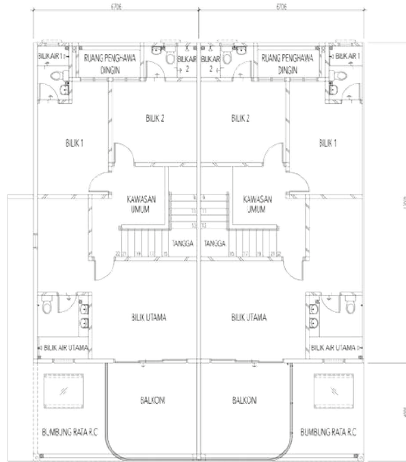
PELAN ARAS 1
