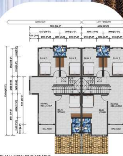
PELAN LANTAI TINGKAT ATAS
