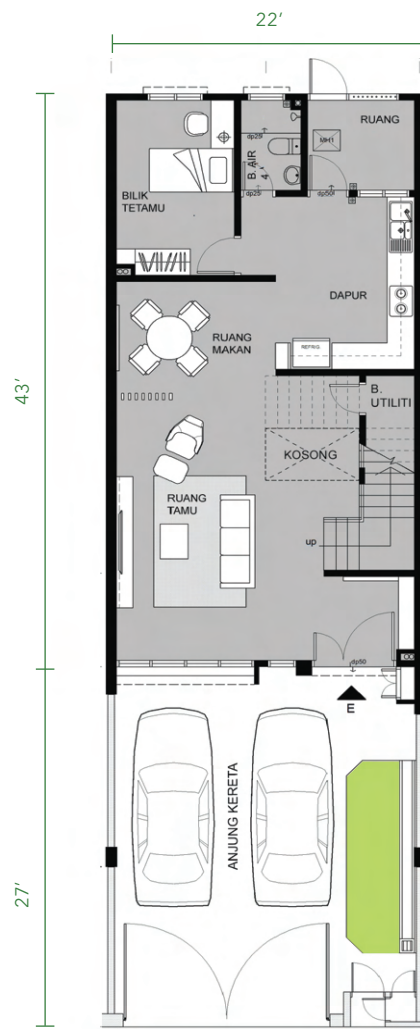
PELAN TINGKAT BAWAH
