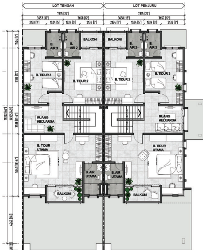
Pelan Tingkat Atas
