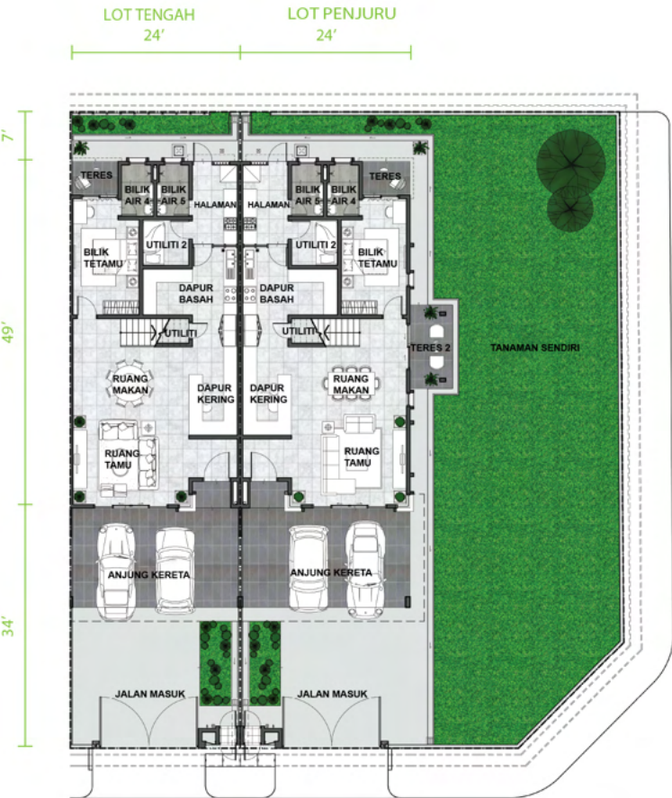
PELAN TINGKAT BAWAH
