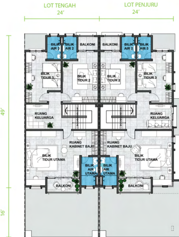
PELAN TINGKAT ATAS
